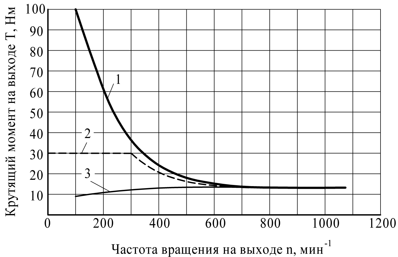
Рис. 4. Нагрузочные характеристики:
